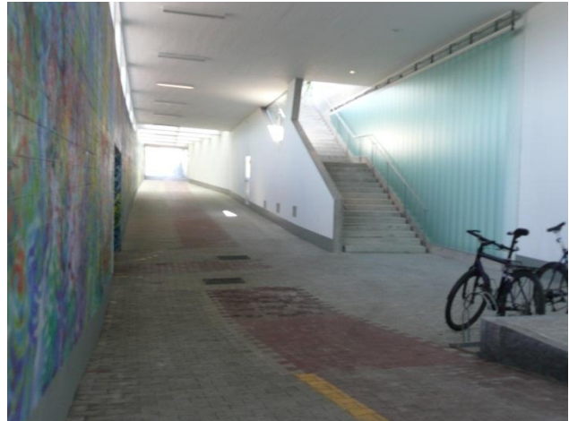
Treppe Richtung Bünishoferstrasse mit LED beleuchteter Profilitverglasung
