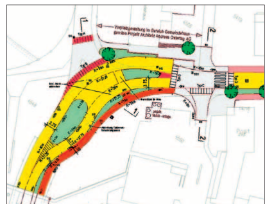
Projektteil Kreuzungsbereich Grütstrasse und Übergang Post/Gemeindehaus
